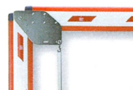
WA14 articulație pentru bare WA1 (de la 1850 mm la 2400 mm)
